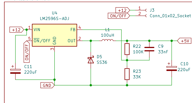
Alimentazione 5 Volt
