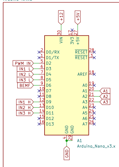
Arduino NANO
