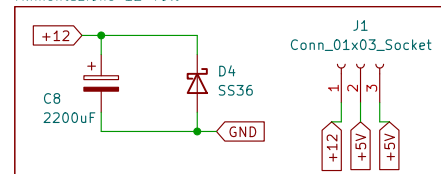
Alimentazione 12 Volt
